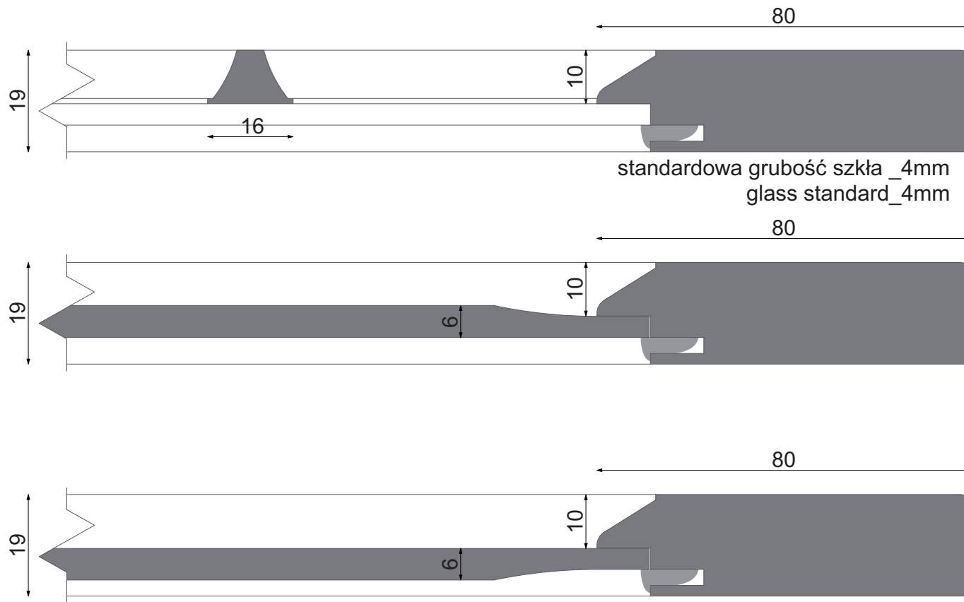
DETAL _ PRZEKRÓJ / DETAIL _ SECTION
