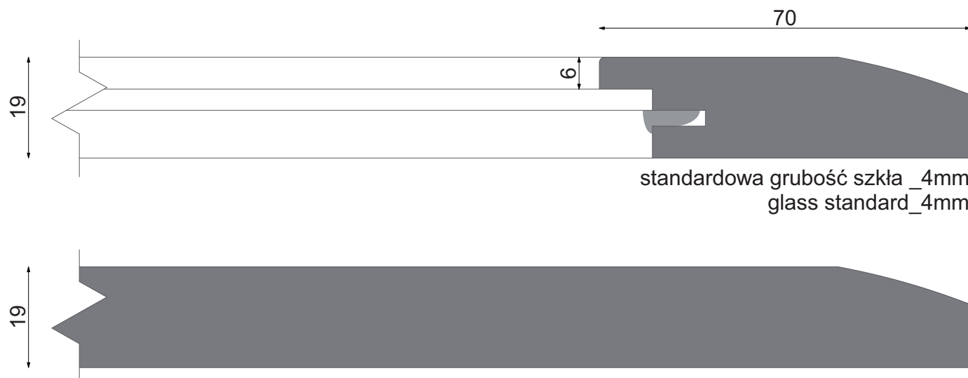
DETAL _ PRZEKRÓJ / DETAIL _ SECTION
