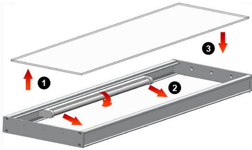
schéma výměny zdroje světla
