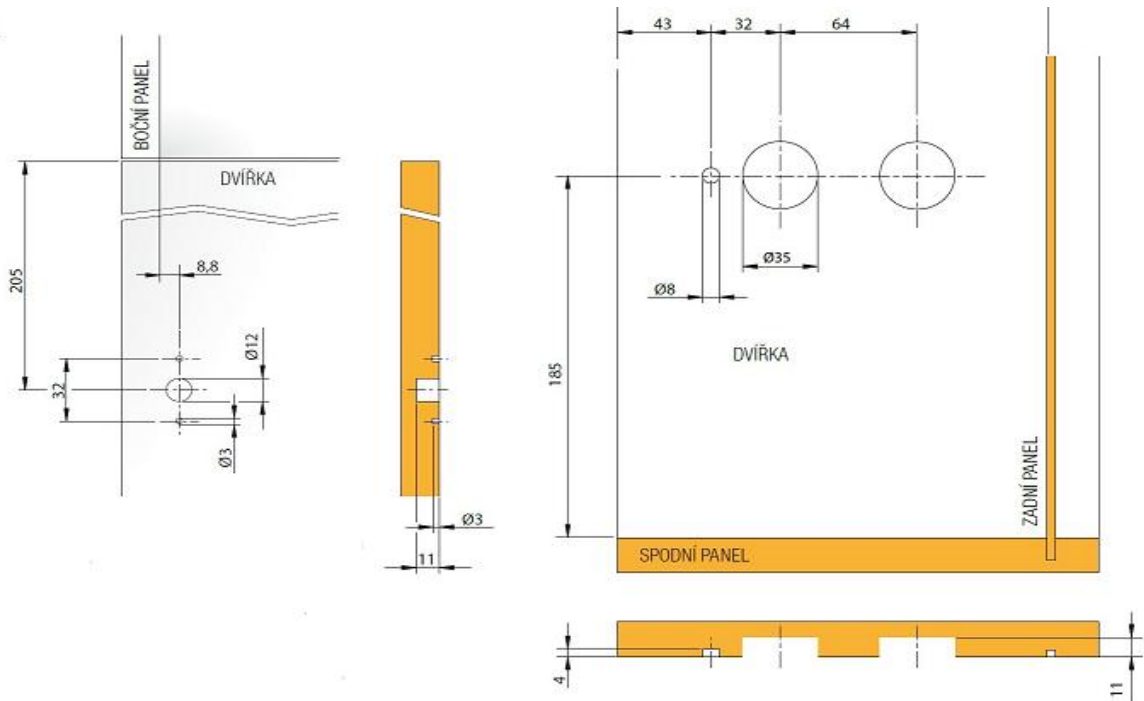
VRTACÍ SCHEMA
