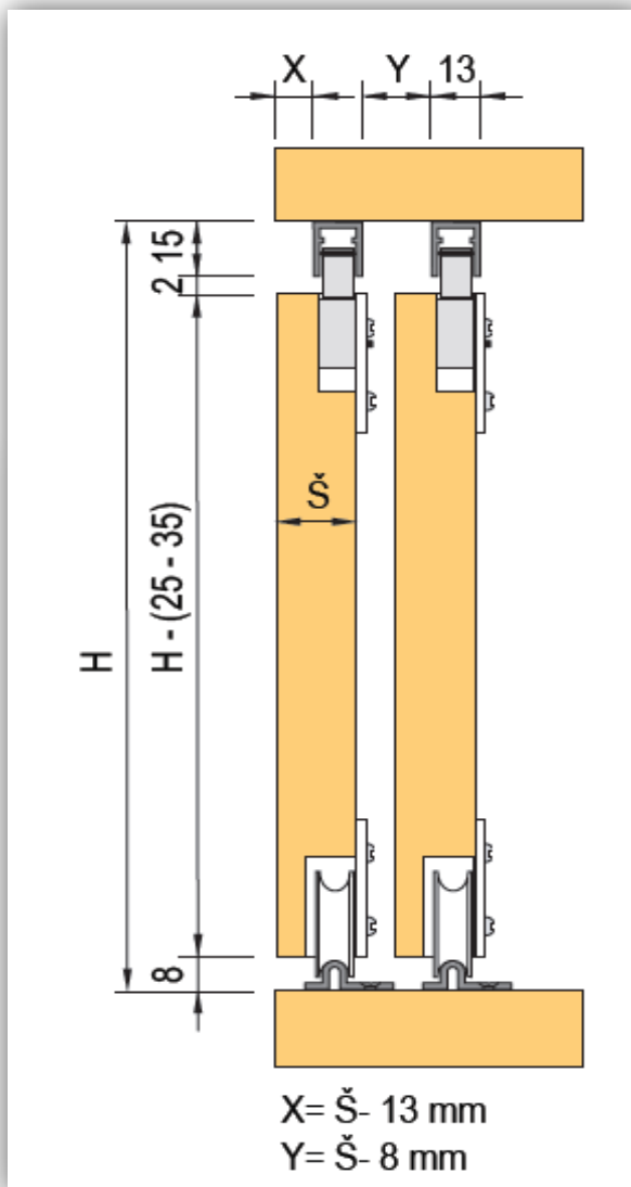
dolní kolej k našroubování
